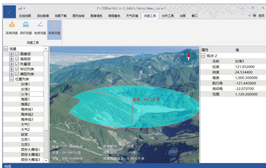
图 10-1 高度测量
